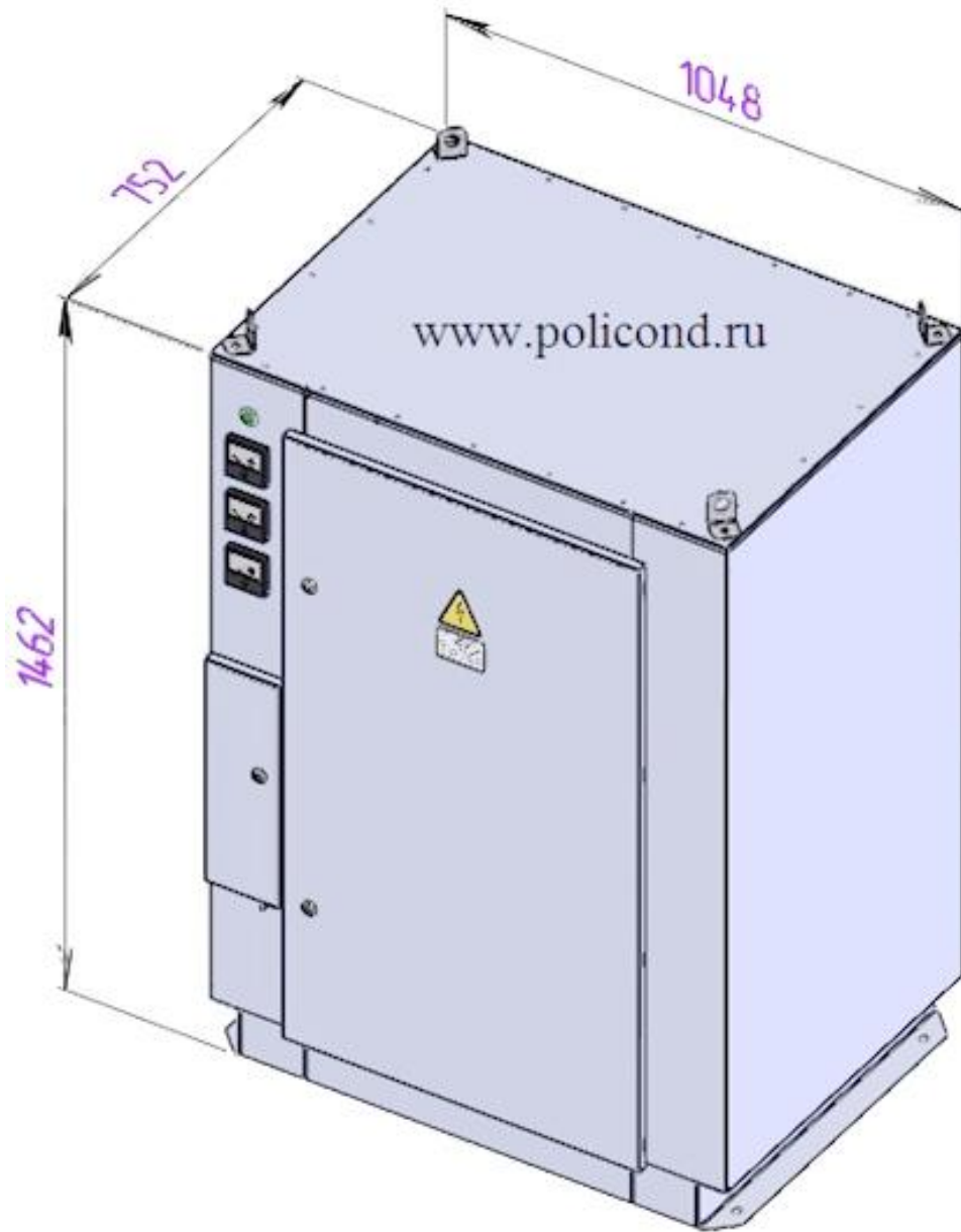
Рис 1. УКЛ56(57)-6,3-(450;600) УЗ
