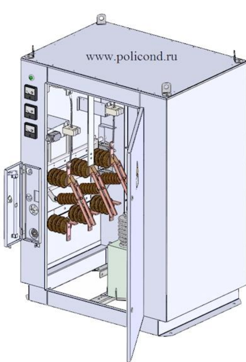
Рис 3. УКЛ56-6,3-450 У3
