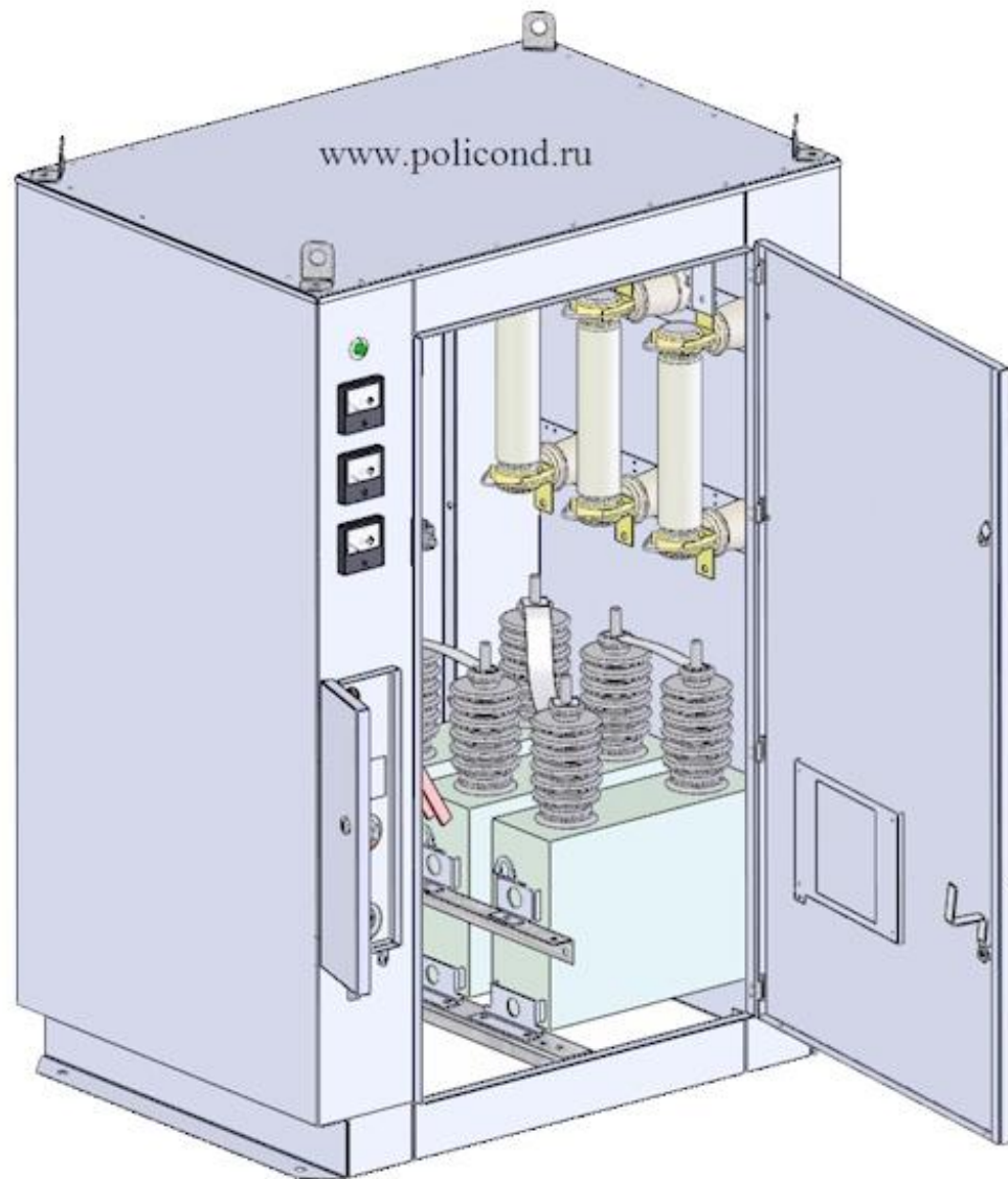
Рис 4. УКЛ56-6,3-450 У3
