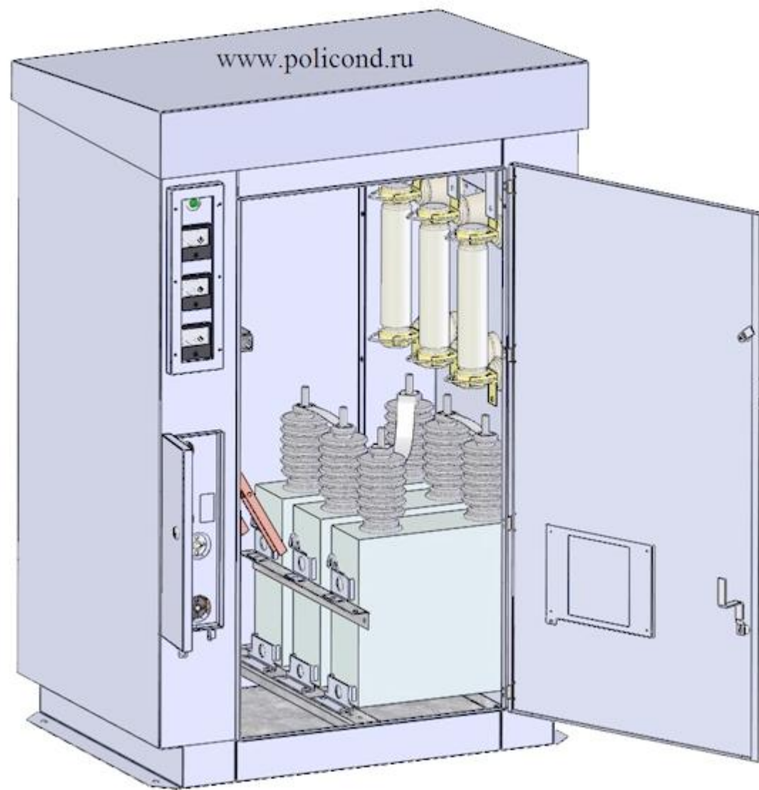
Рис 4. УКЛ156-6,3-600 У1
