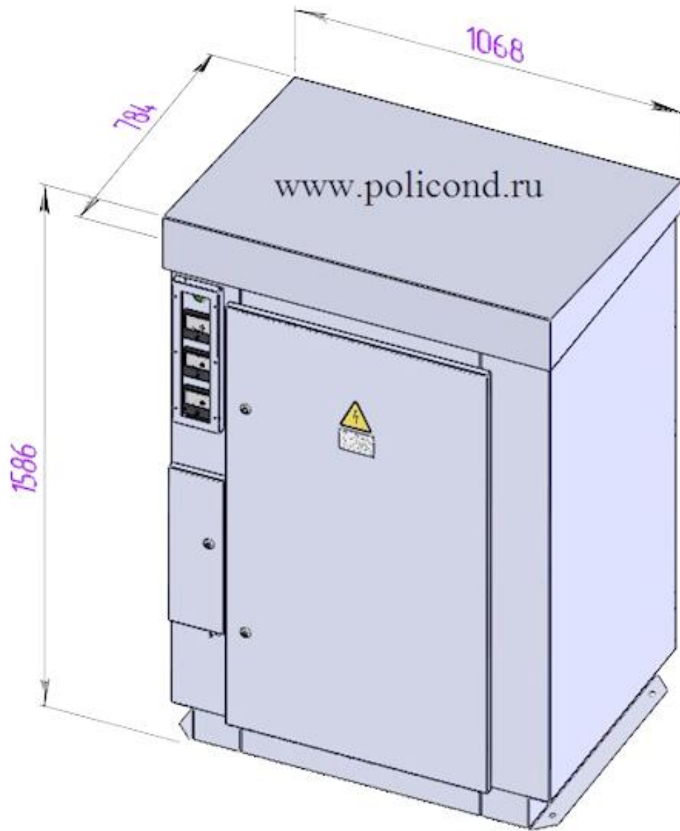
Рис 1. УКЛ56(57)-6,3-(450;600) У1
