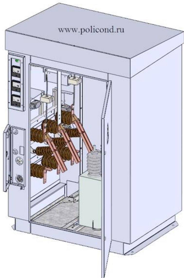
Рис 3. УКЛ156-6,3-600 У1
