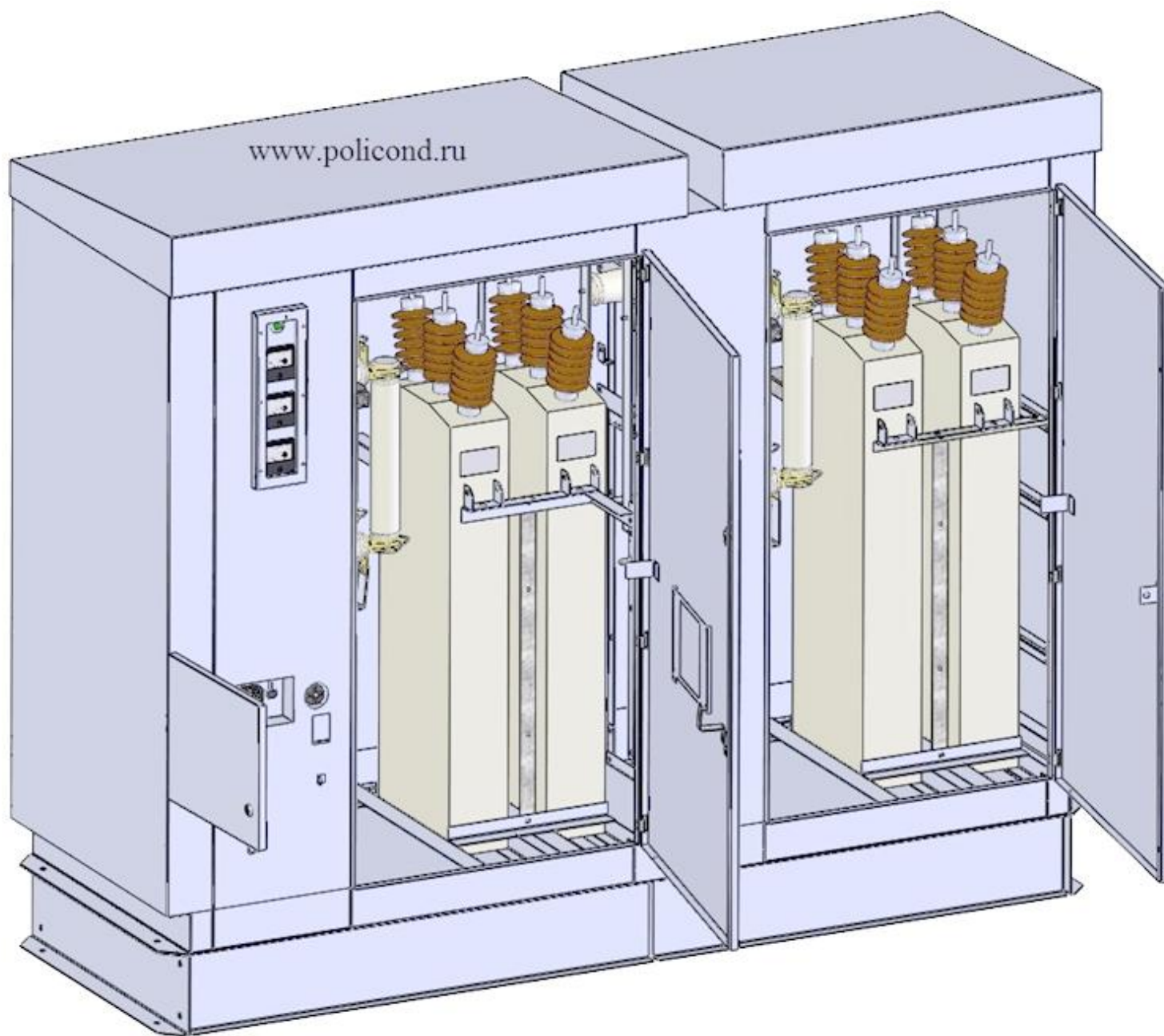
Рис 4. УКЛ56(57)-10,5-1800 У1
