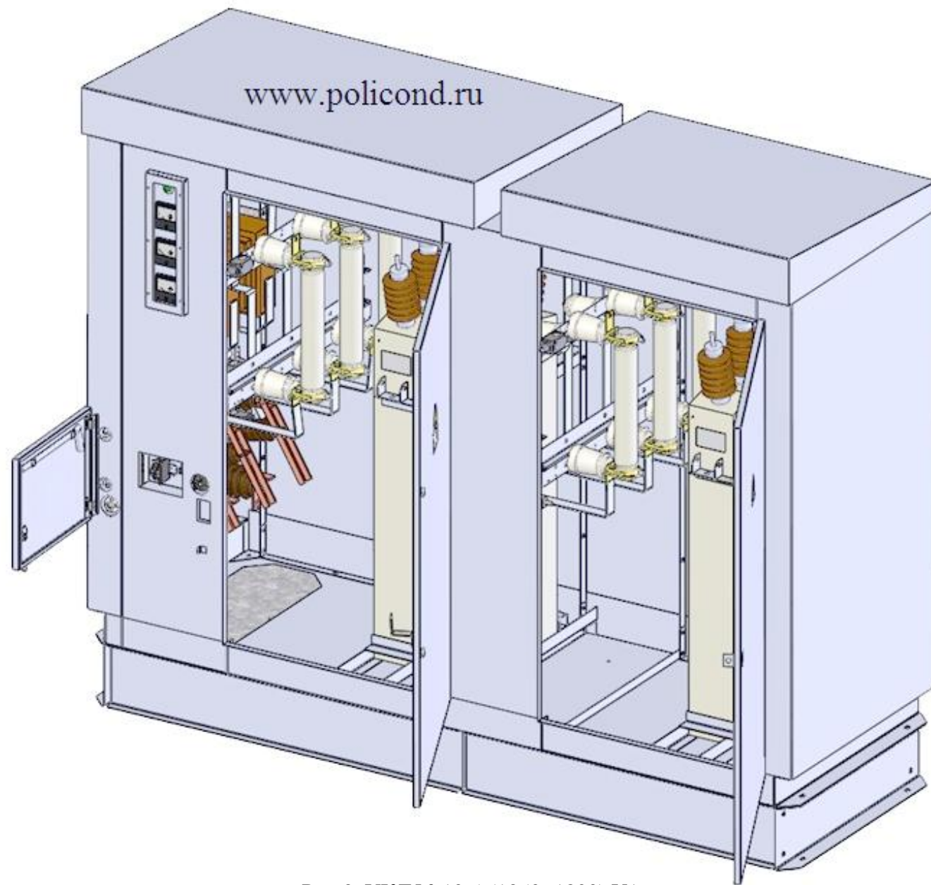
Рис 3. УКЛ56-10,5-(1350÷1800) У1
