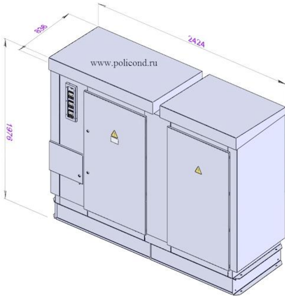
Рис 1. УКЛ56(57)-10,5(6,3)-(925÷1800) У1
