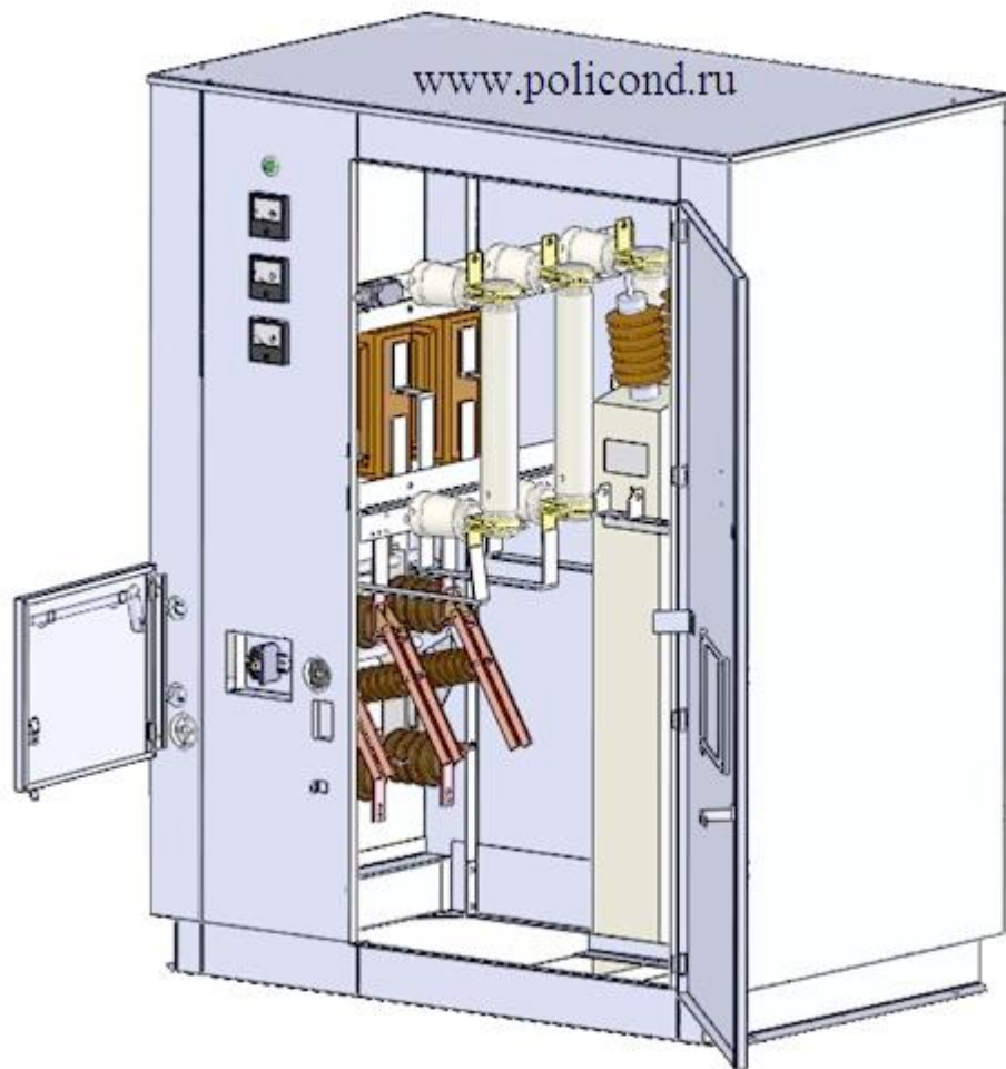
Рис 3. УКЛ156-10,5-900 У3
