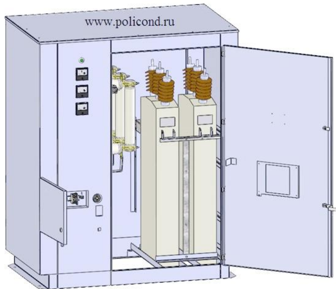
Рис 4. УКЛ156-10,5-900 У3
