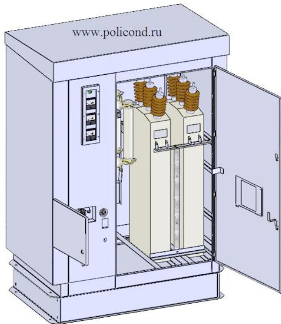
Рис 4. УКЛ156-10,5-900 У1
