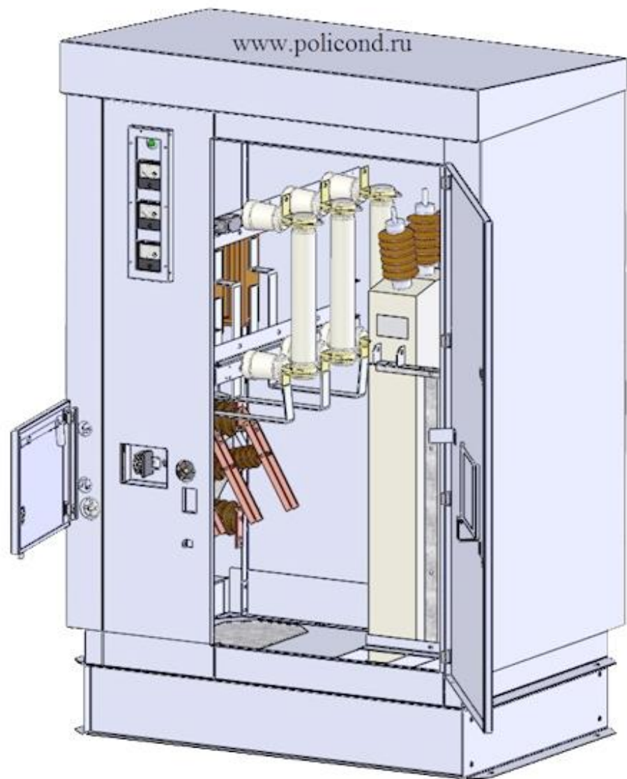
Рис 3. УКЛ156-10,5-900 У1
