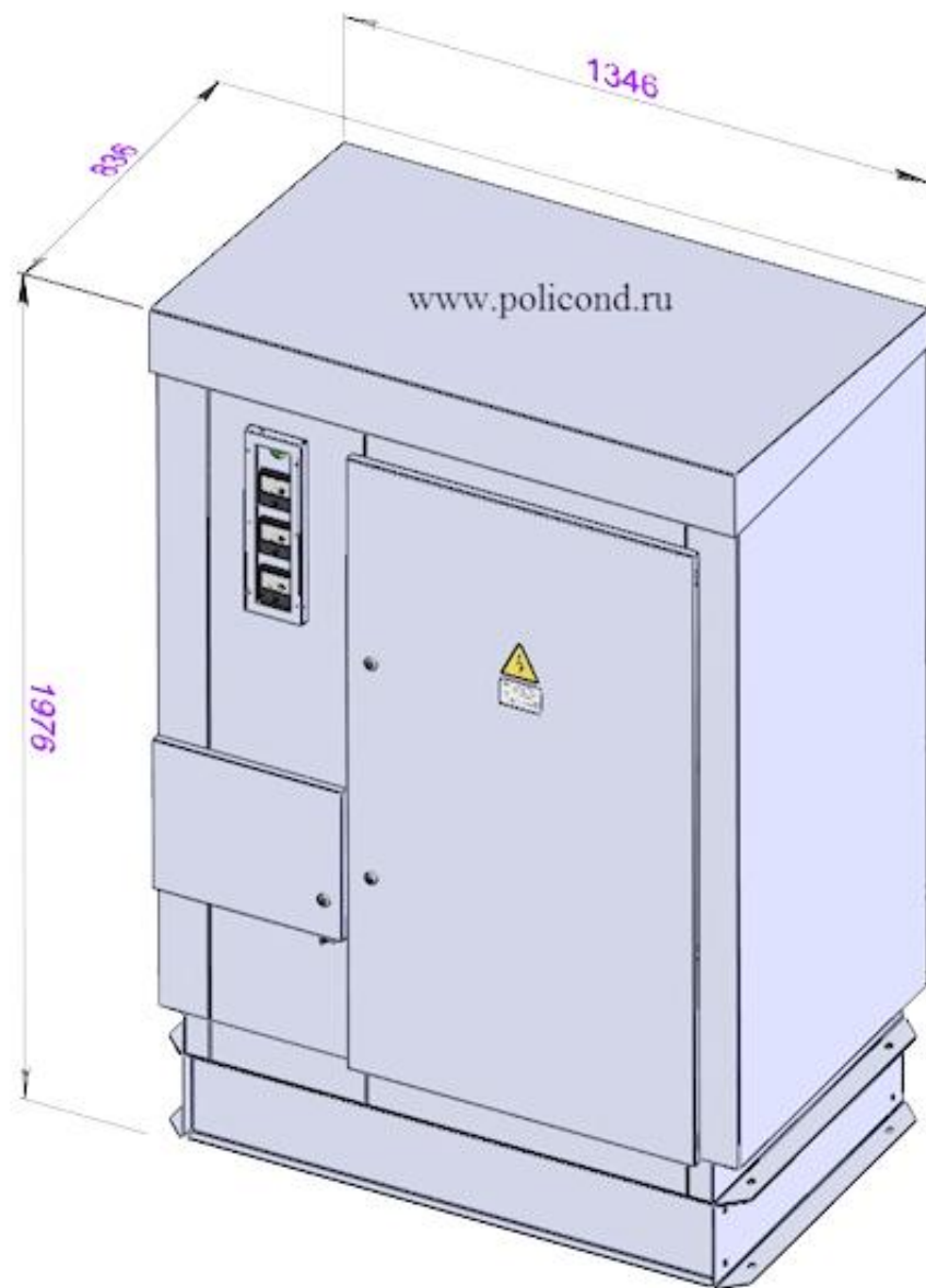
Рис 2. УКЛ56(57)-10,5(6,3)-(25÷900) У1
