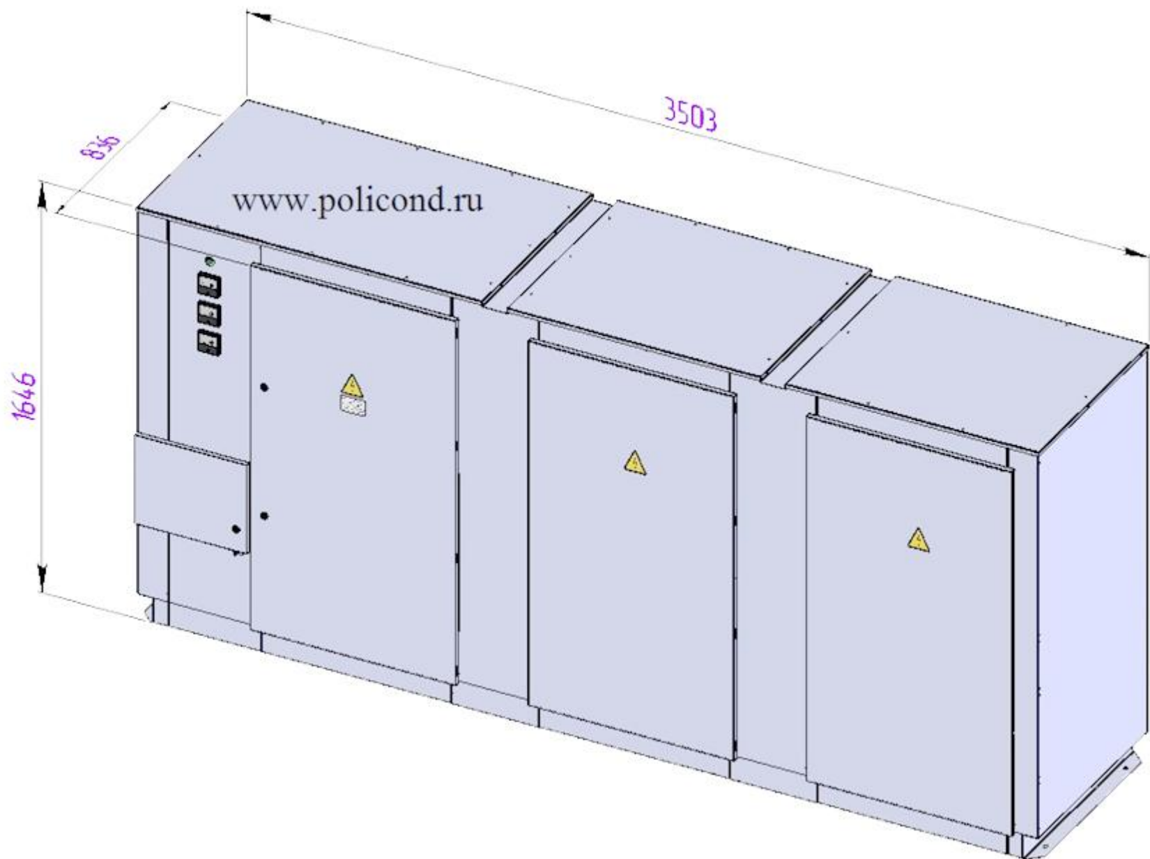
Рис 1. УКЛ56(57)-10,5(6,3)-(1925÷2700) У3
