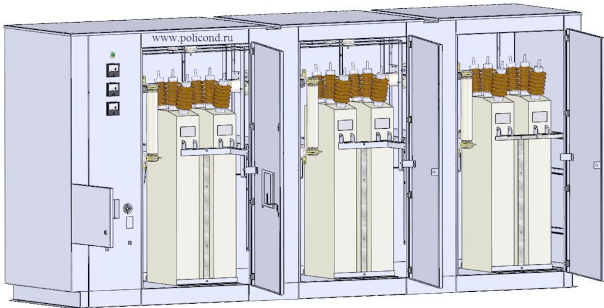
Рис 4. УКЛ56-10,5-2700 У3
