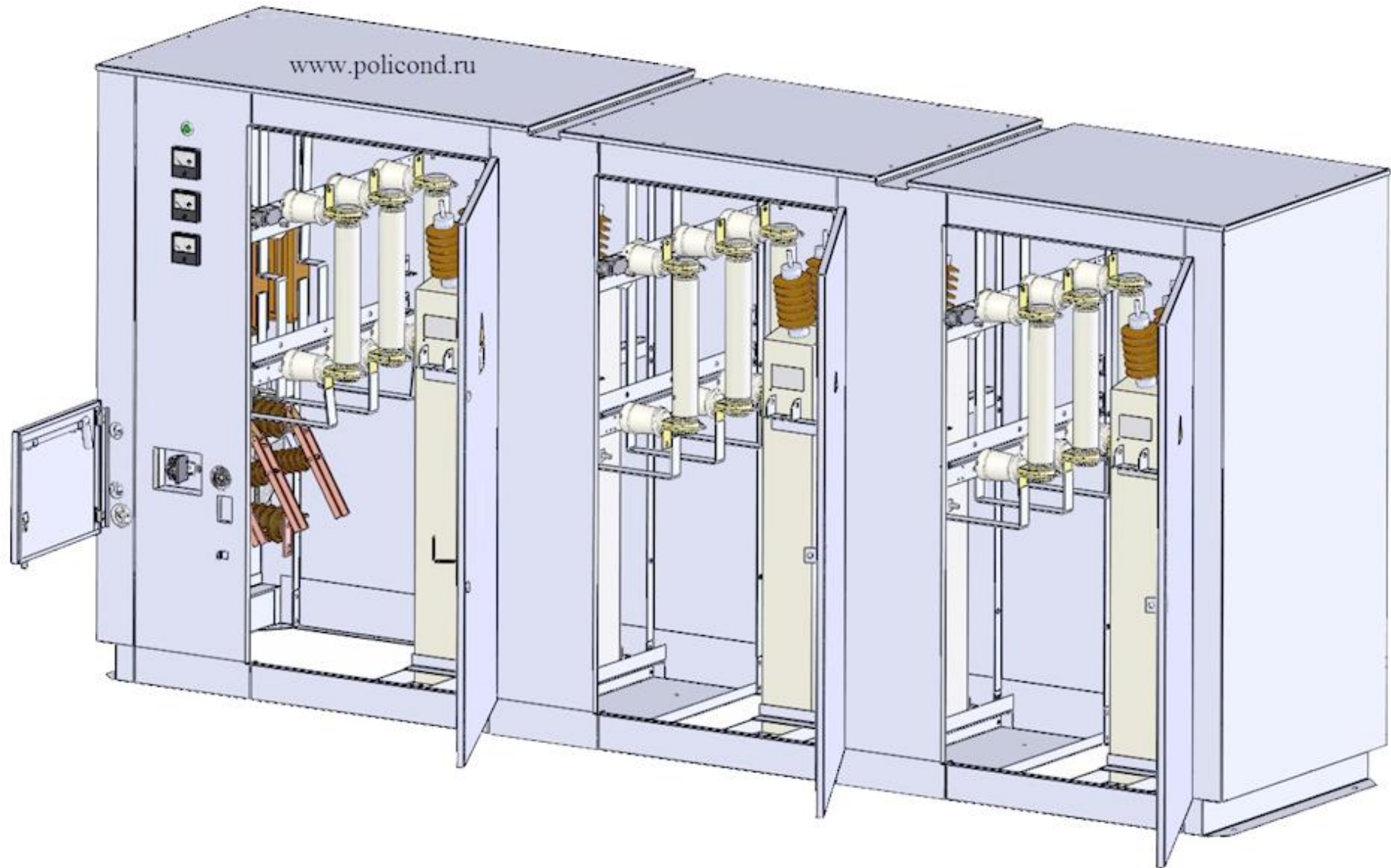
Рис 3. УКЛ56-10,5-2700 У3
