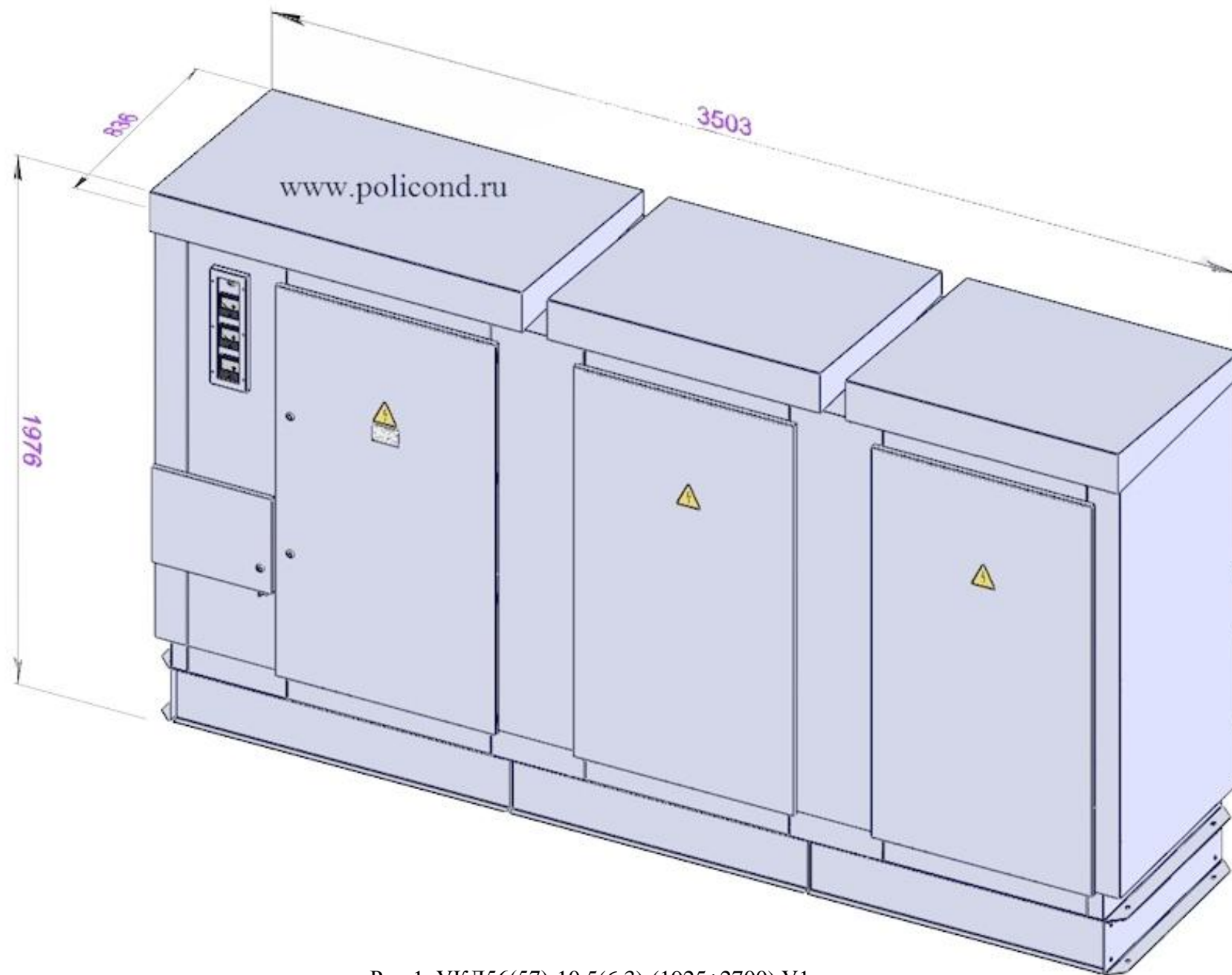
Рис 1. УКЛ56(57)-10,5(6,3)-(1925÷2700) У1
