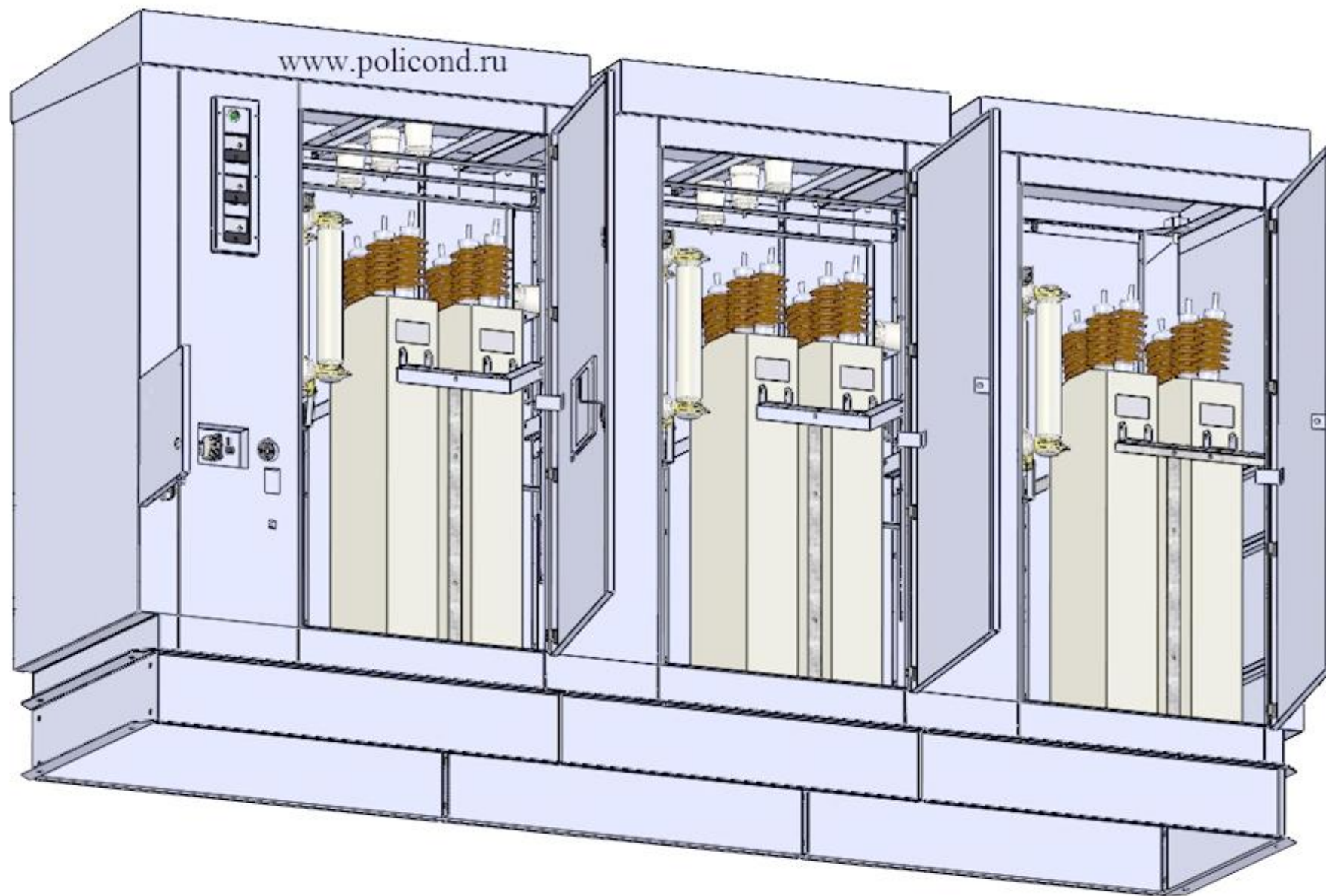
Рис 4. УКЛ56-10,5-2700 У1
